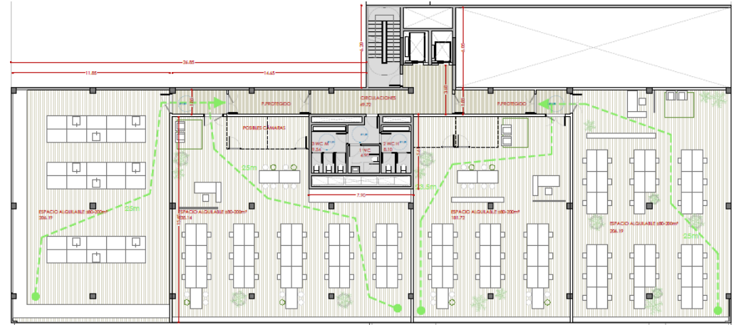
*Planta Tipo: Planta 1ª
