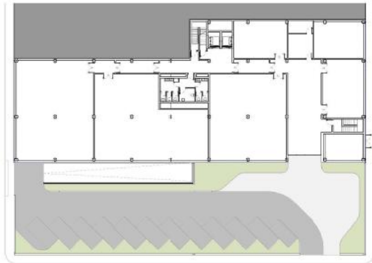
*Planta Tipo: Planta Baja
